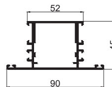
DOOR MULLION CODE - C0M02M WEIGHT KG/M - 1.460
