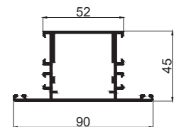
DOOR MULLION CODE - C0M02M WEIGHT KG/M - 1.460
