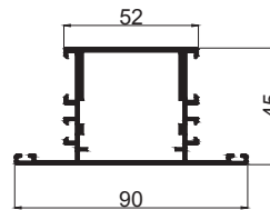
DOOR MULLION CODE - C0M02M WEIGHT KG/M - 1.460
