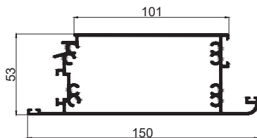
DOOR BOTTOM SECTION CODE - CM09BM WEIGHT KG/M - 2.422
