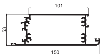
DOOR BOTTOM SECTION CODE - CM09BM WEIGHT KG/M - 2.422
