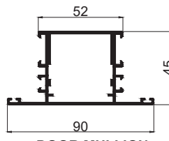
DOOR MULLION CODE - C0M02M WEIGHT KG/M - 1.460
