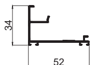
DOOR BOTTOM CLIP CODE - CM09CM WEIGHT KG/M - 0.542
