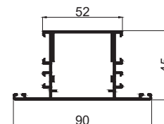
DOOR MULLION CODE - C0M02M WEIGHT KG/M - 1.460
